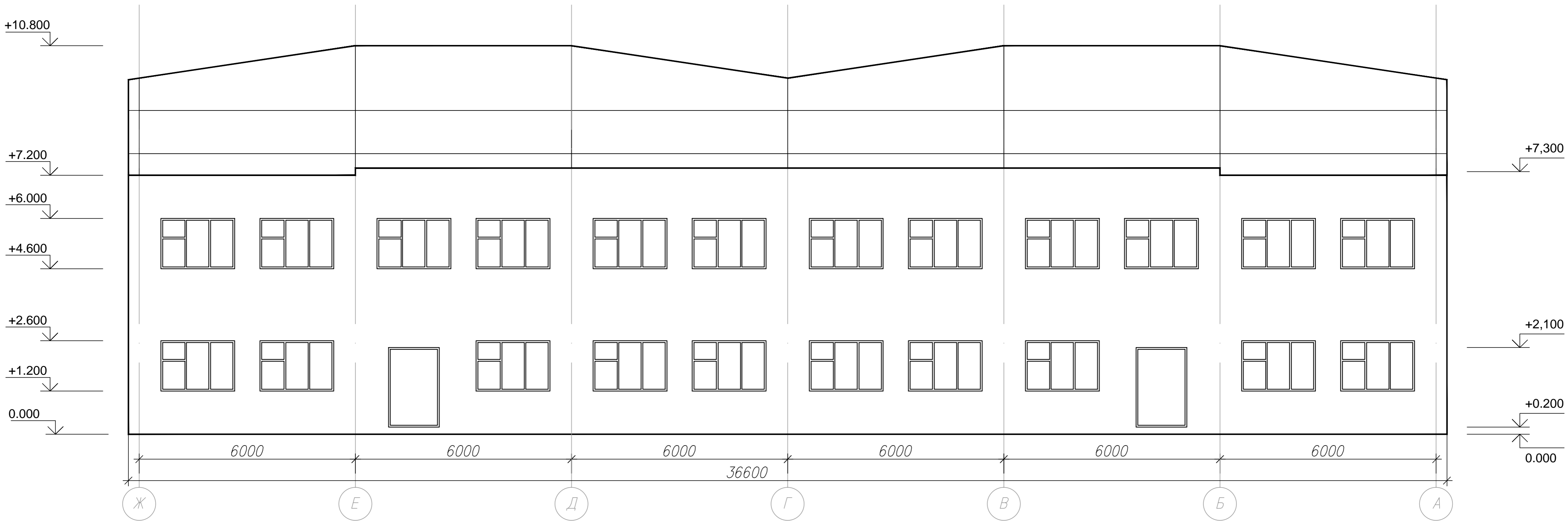
План фасада по оси 3'/Ж-А
